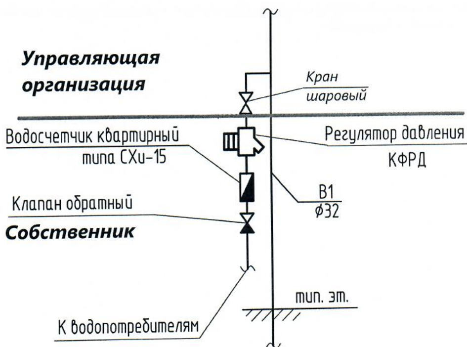
Схема ХВС
